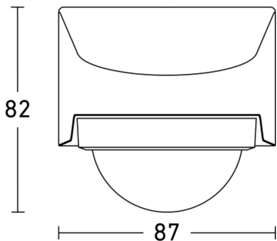
Dessin dimensionnel 1
